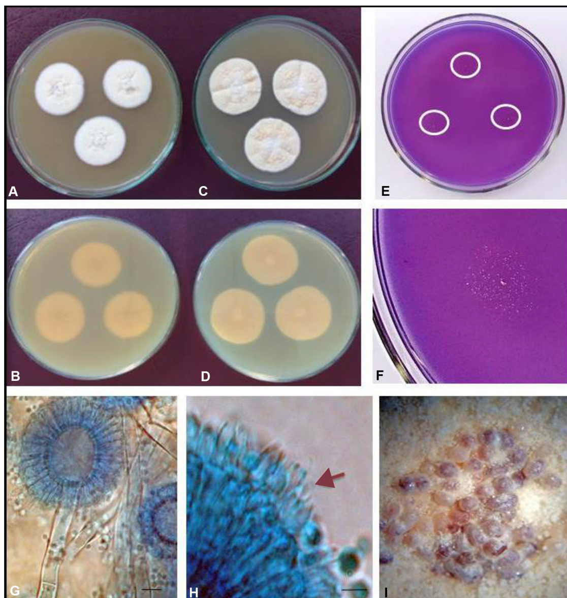
Figura 1 A,B) MEA (anverso, reverso) 25 °C. C,D) CYA 25 °C. E,F) CREA (anverso) 25 °C. En círculo, los puntos de crecimiento poco visibles. F) Detalle del escaso crecimiento a gran aumento. G) Conidióforo, métulas, fialides y conidios. H) Gran aumento de métulas y fialides. I) Esclerocios en CYA.
